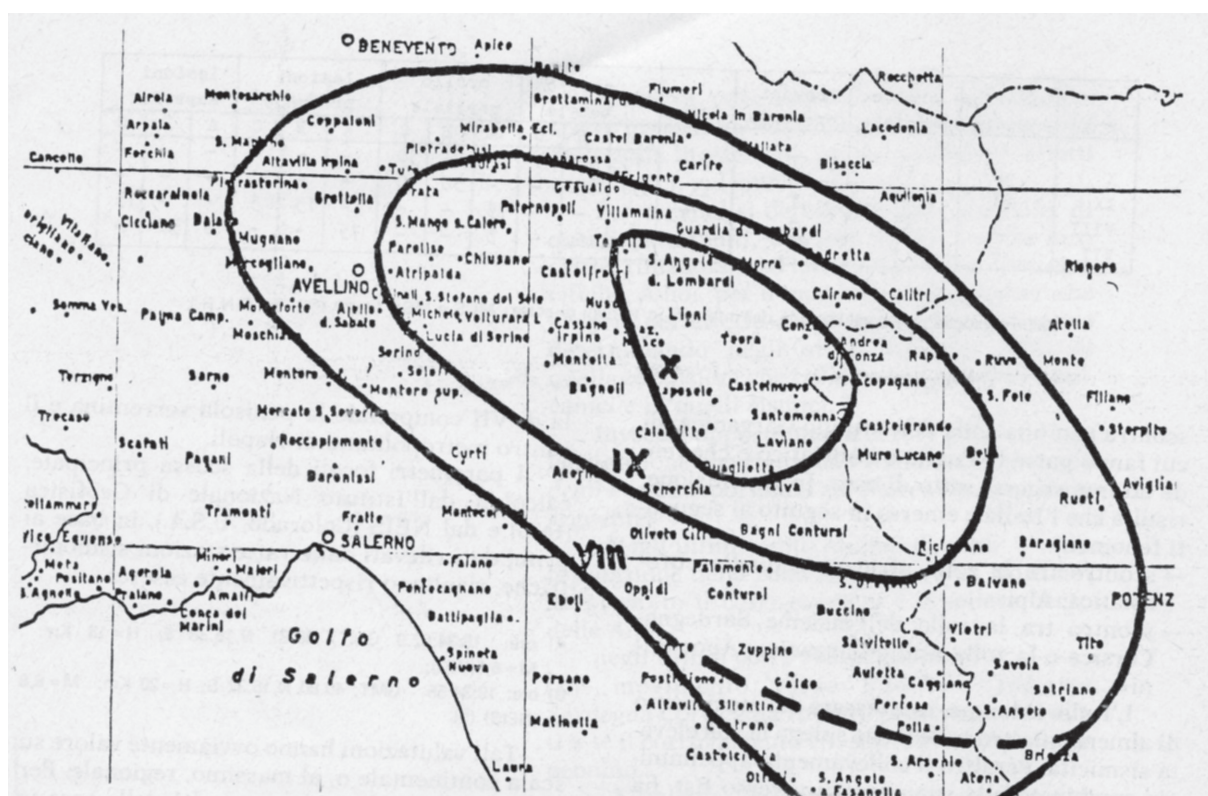
Fig. 7: Terremoto del 23 - XI - 1980 - Mappa sismica in scala MCS
