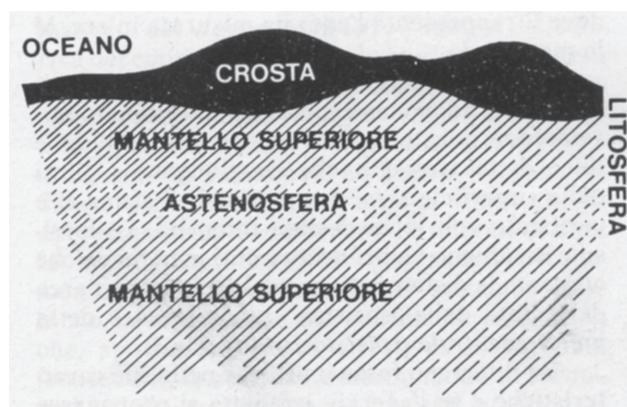
Fig. 4: L'interno della Terra nei primi 400 Km circa
