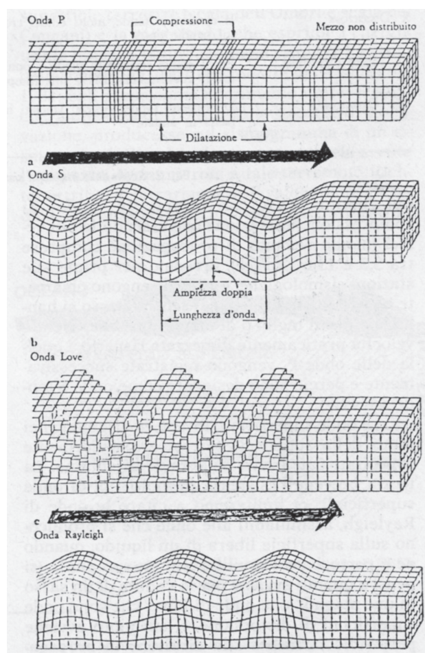
Fig. 1 : I vari tipi di onde sismiche
