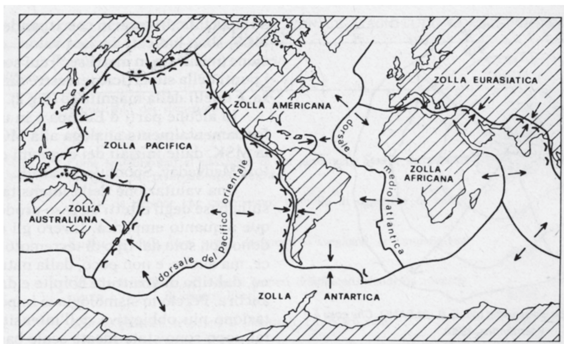
Fig. 5: Le principali zolle crostali - Le frecce indicano la direzione dei movimenti
