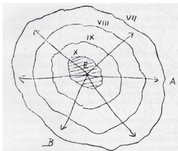
Fig. 3: Sistema di linee isosismiche
